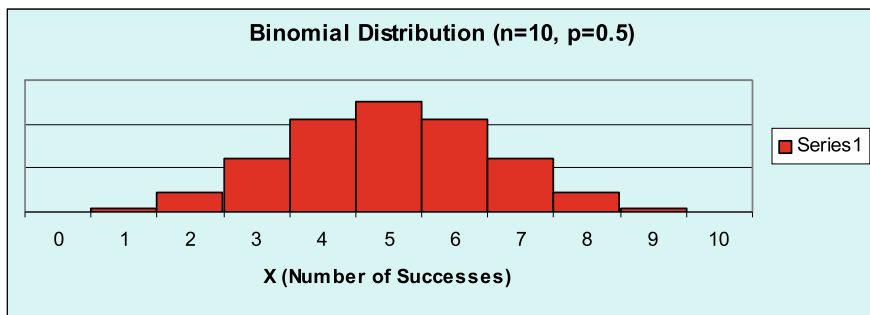
Fig. 23.1 Binomial distribution
